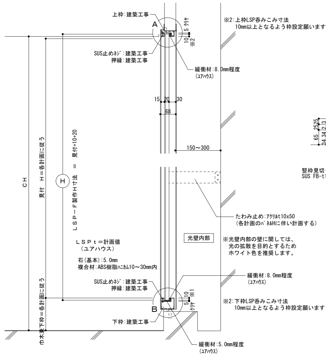
断面詳細図 1/10
